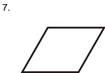
Rhombus
