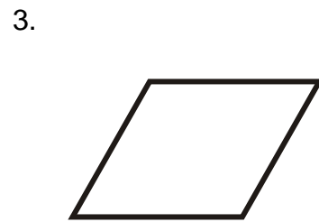
Rhombus
